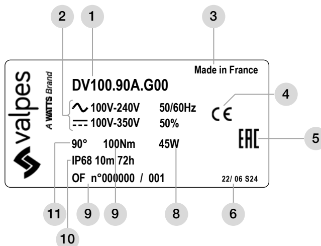
Plaque d'identification (extérieur - carter)
